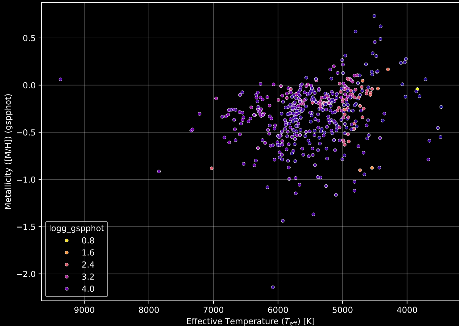
GALAH DR4 Field: [6592] Stellar Population Parameters (n= 453)
